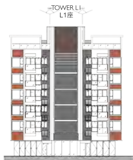
ELEVATION G - TOWER LI 立面圖 G - L1座
